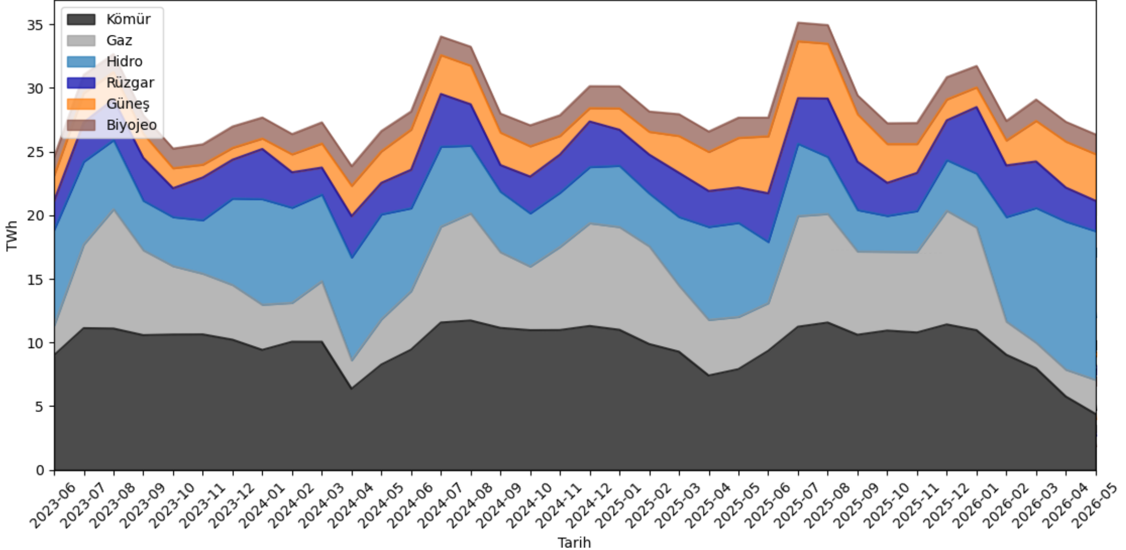
Kaynaklara Göre Elektrik Üretimi - Son 36 Ay
