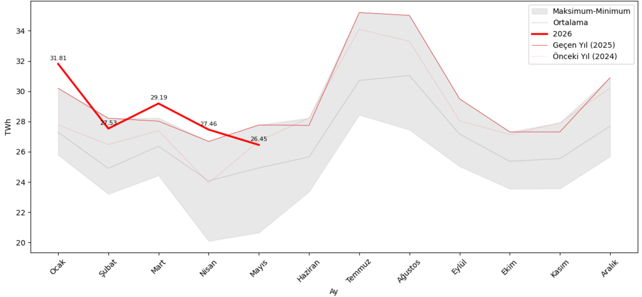
Elektrikte Aylık Üretim - Toplam Üretim
