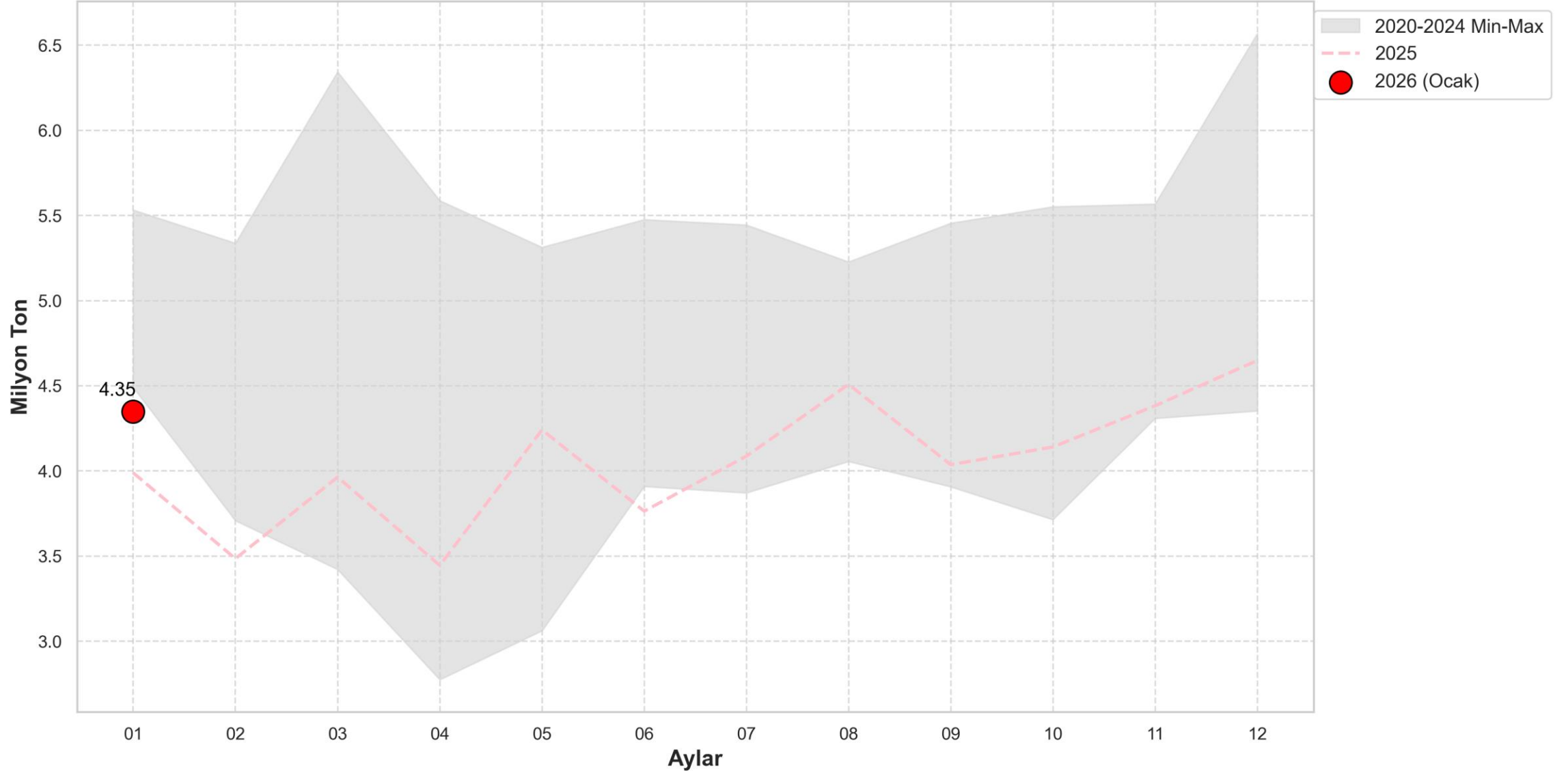
Linyit - (Elektrik) Aylık Gelişim ve 2026
