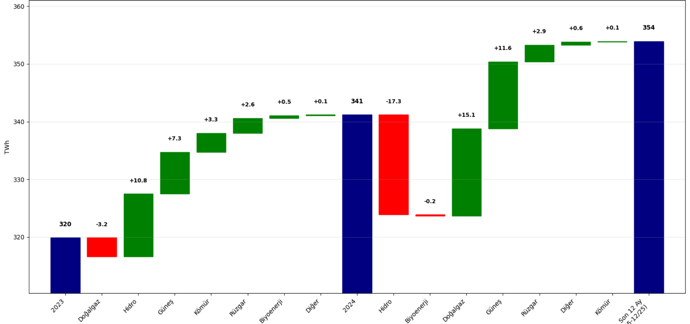
Türkiye Elektrik Üretimi Değişimi
