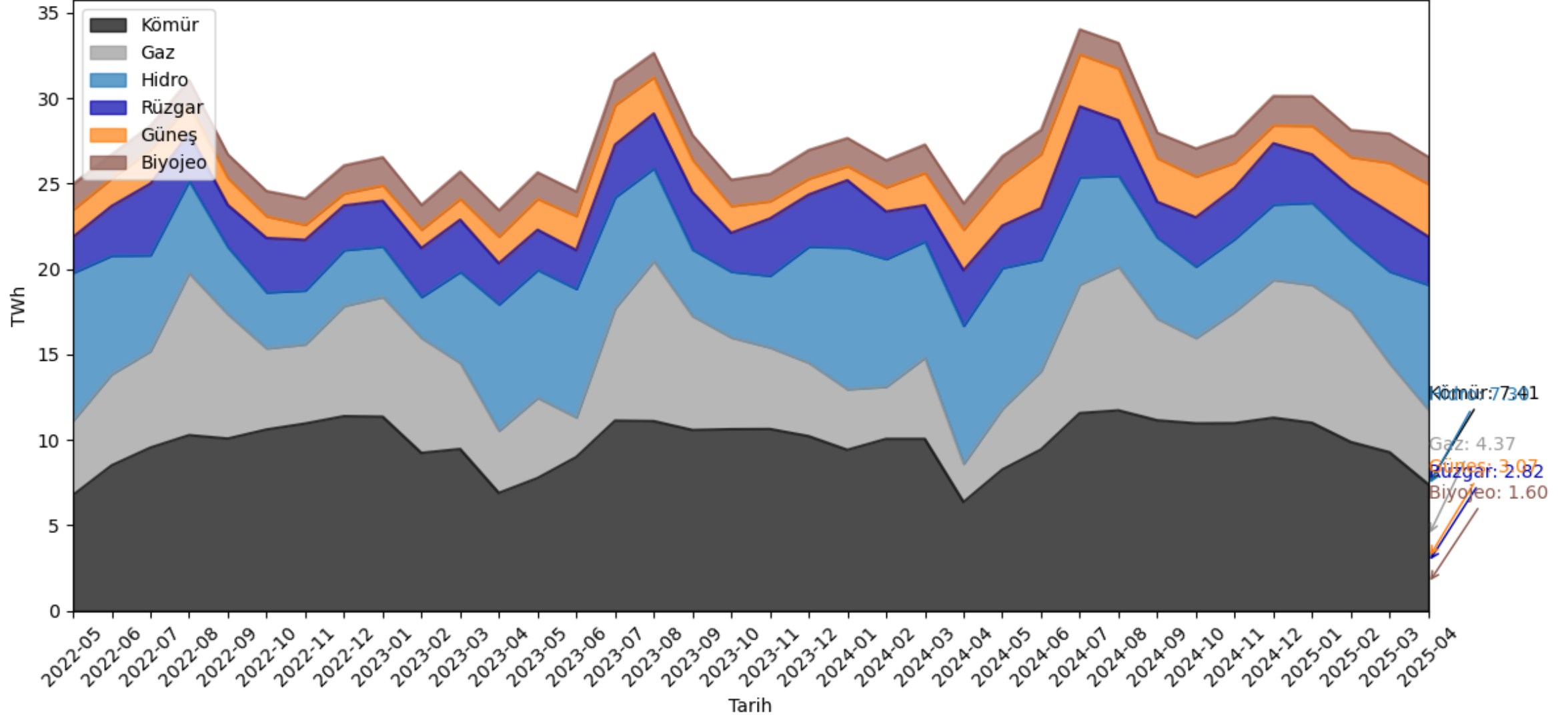
Kaynaklara Göre Elektrik Üretimi - Son 36 Ay
