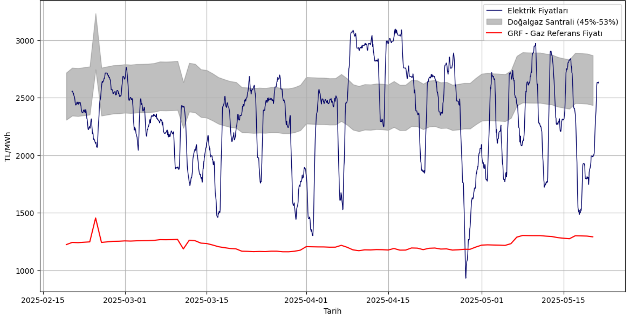
Elektrik Fiyatları (24 Saat Ortalama), Doğalgaz Santrali (%45-53), GRF Gaz Fiyatı
