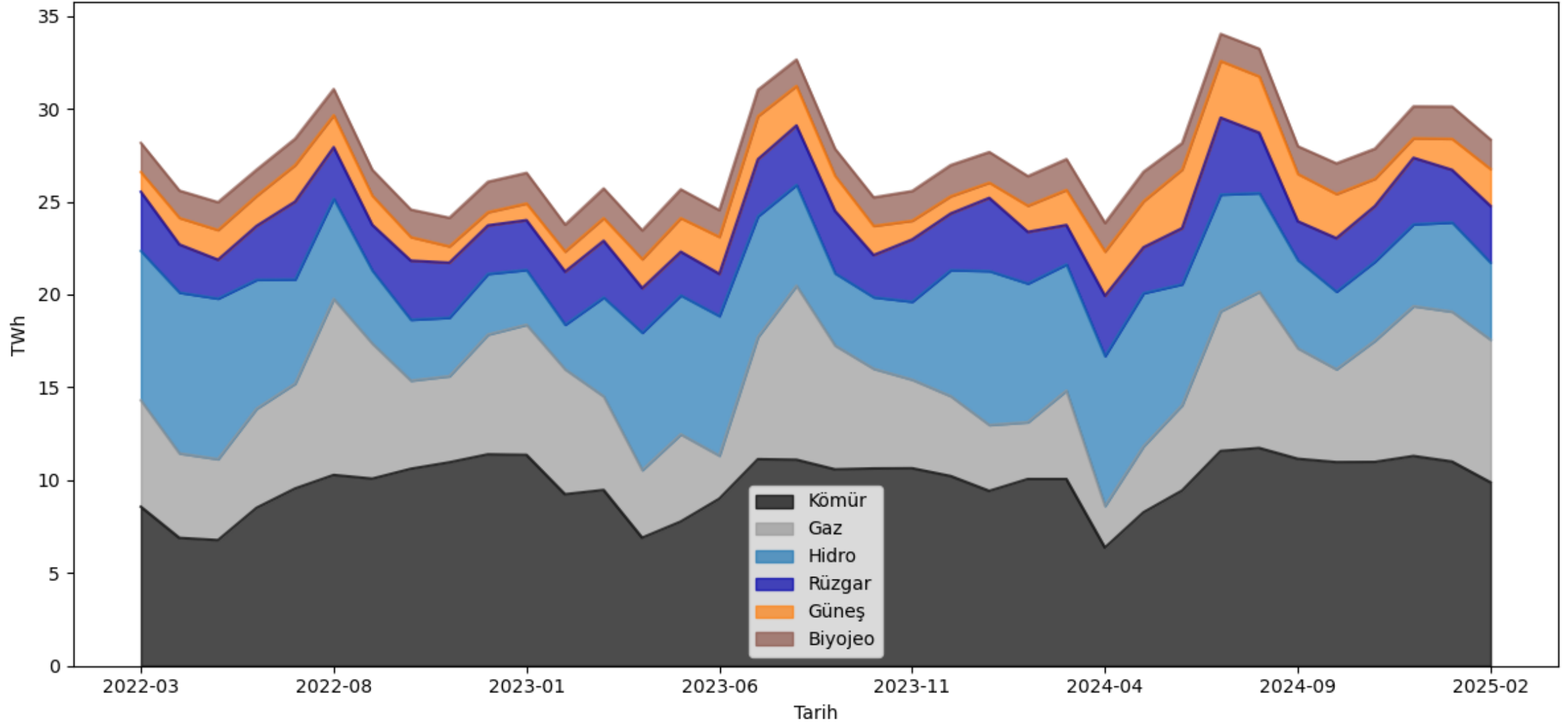
Kaynaklara Göre Elektrik Üretimi - Son 36 Ay
