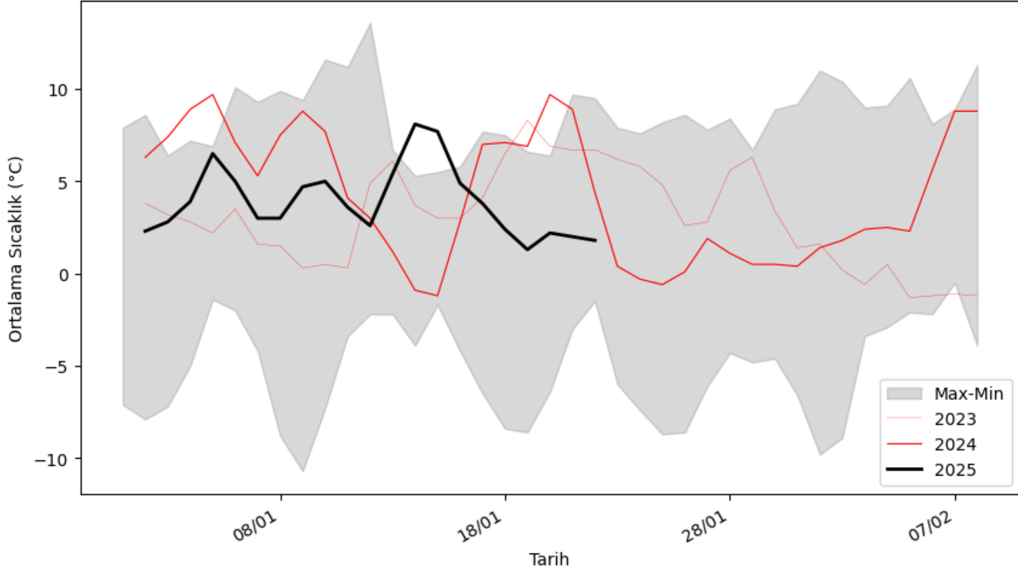
Günlük Ortalama Sıcaklıklar
